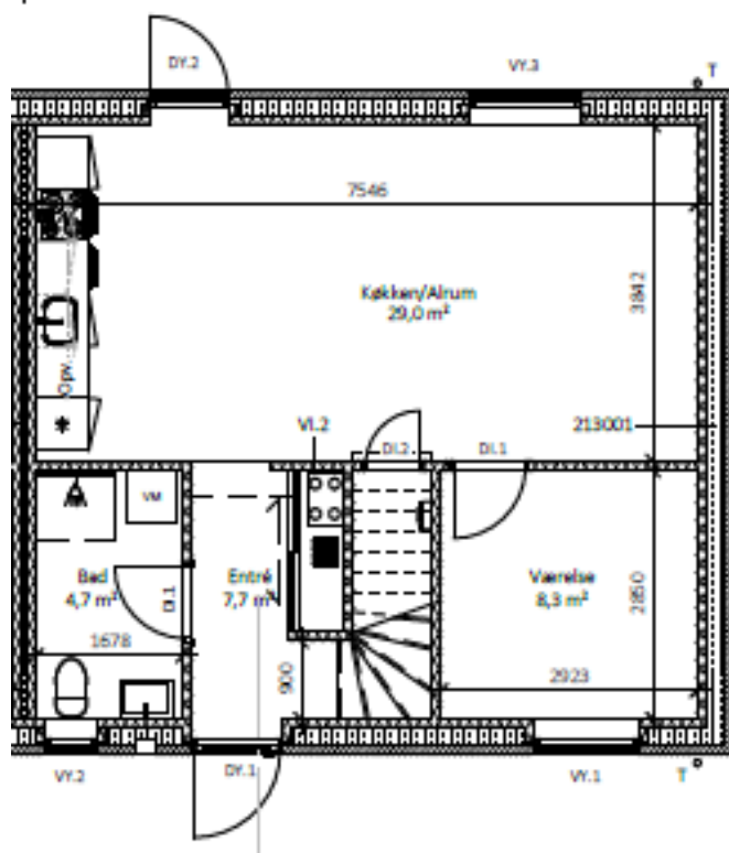
Stueplan
